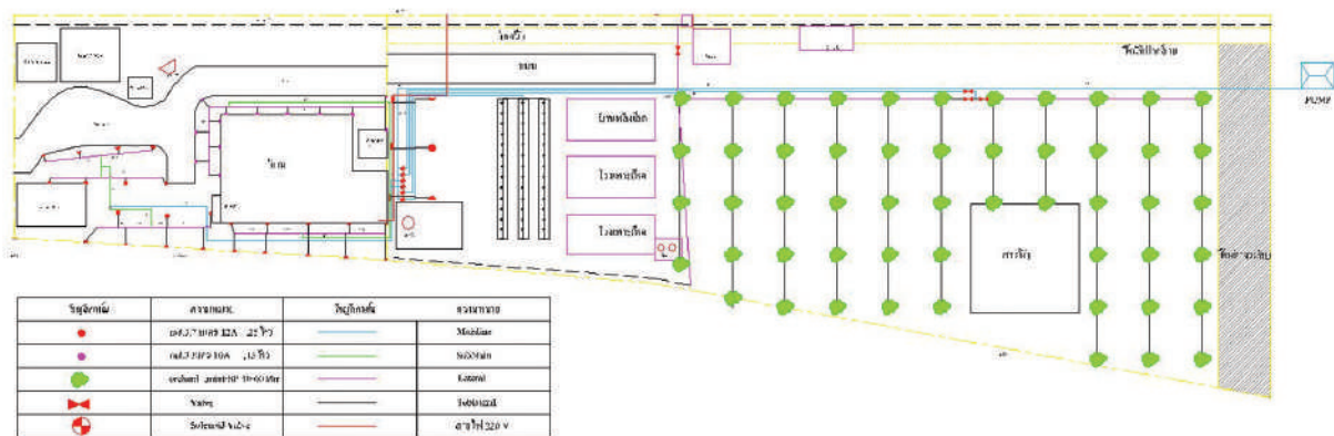
แบบแปลนระบบน้ำอัตโนมัติ
