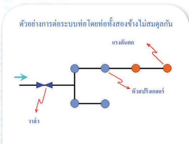
ภาพที่ 67 ตัวอย่างการวางแนวท่อที่ไม่สมดุลและการวางแนวท่อให้สมดุล
