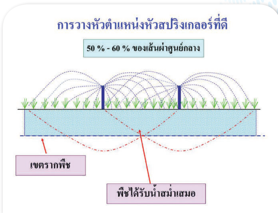
ภาพที่ 19 การซ้อนทับของวงน้ำที่วางหัวได้ระยะที่เหมาะสมทำให้พื้นที่ได้รับน้ำสม่ำเสมอ
