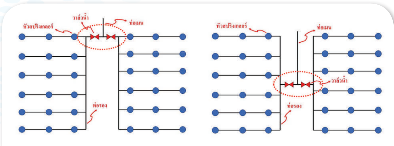
ภาพที่ 24 ตัวอย่างการวางแผนท่อเมนเข้าระบบที่ไม่สมดุลและการวางแผนท่อให้สมดุล
