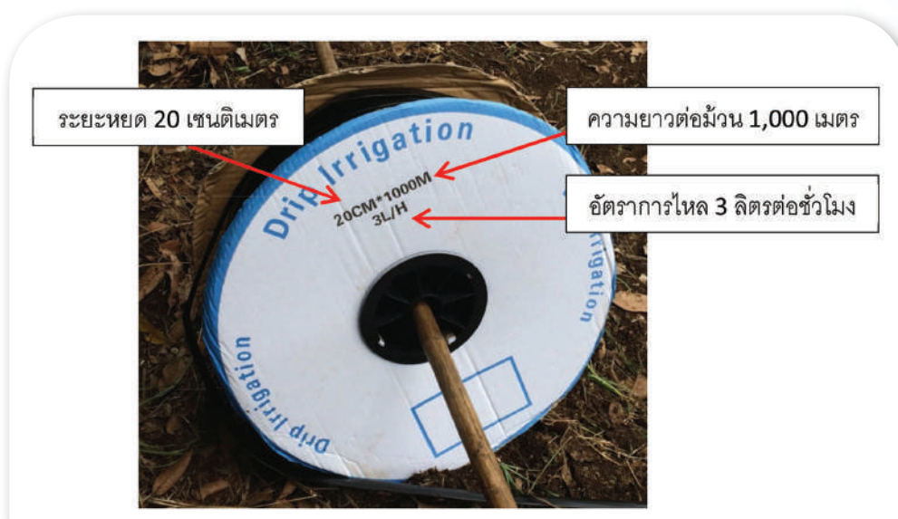
ภาพที่ 55 ป้ายแสดงข้อมูลทางเทคนิคของเทปน้ำหยดที่ติดอยู่ข้างม้วนเทป
