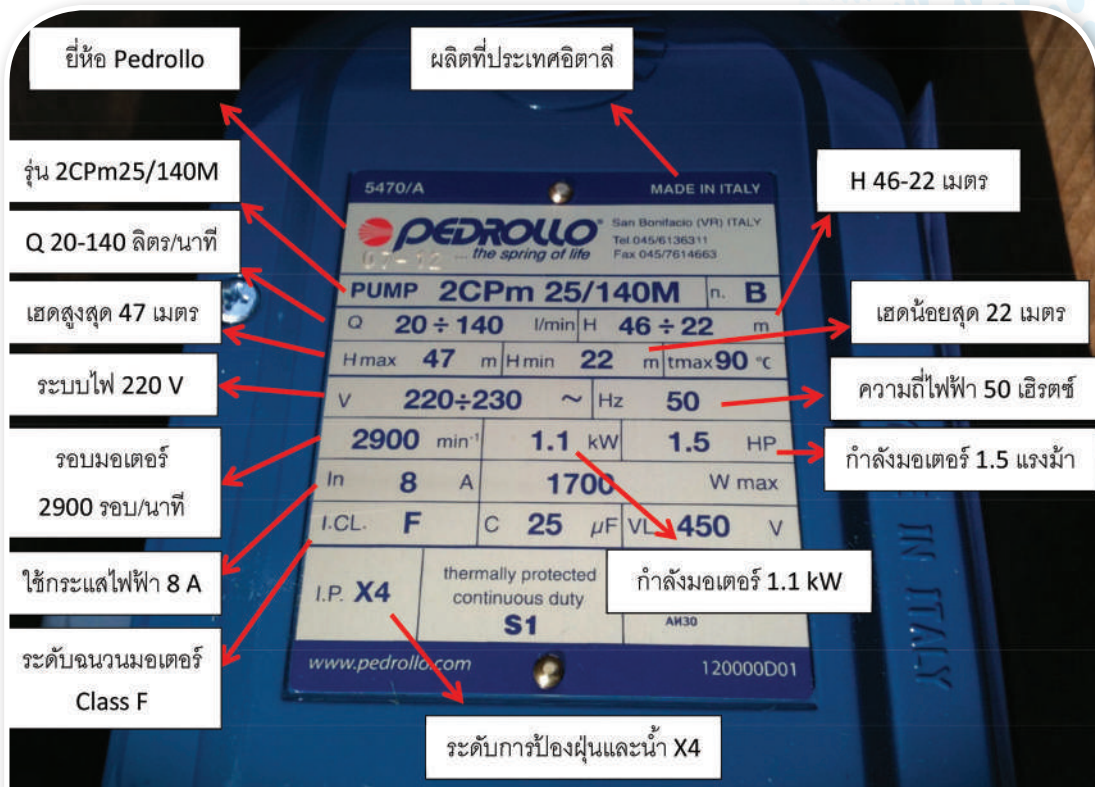
รูปที่ 75 สัญลักษณ์และค่าต่างๆ ในเนมเพลท
