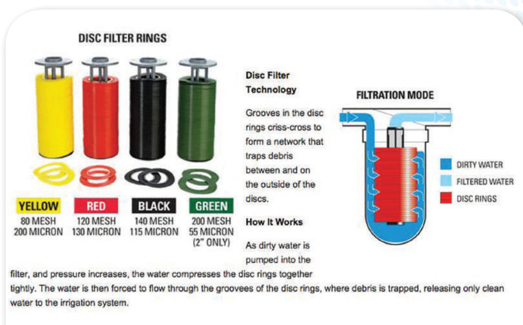
ภาพที่ 42 ใส้กรองเกสรแบบแผ่น และลักษณะการกรองน้ำของกรองชนิดแผ่น ที่มาภาพ https://www.sprinklersupplystore.com/Netafim-Disc-Filters-s/607.htm
