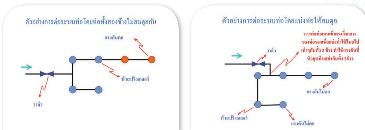
ภาพที่ 23 ตัวอย่างการวางแนวท่อที่ไม่สมดุลและการวางแนวท่อให้สมดุล
