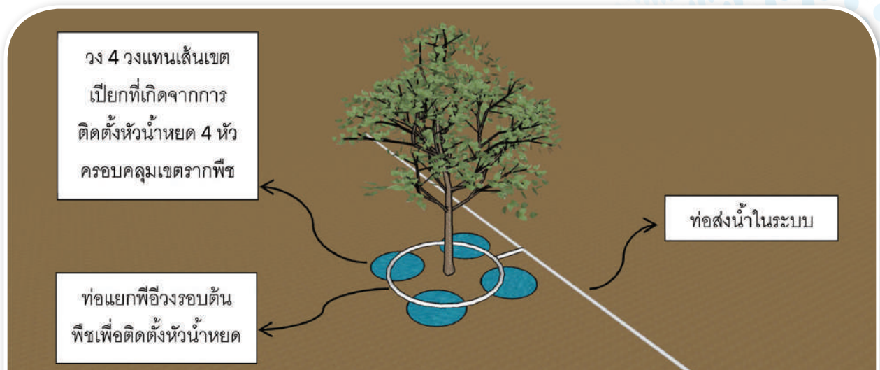
ภาพที่ 62 ตัวอย่างการติดตั้งหัวน้ำหยดสำหรับไม้ยืนต้นโดยใช้วิธีต่อท่อพีอีจนเป็นวงกลมรอบต้นไม้ เพื่อให้สามารถติดตั้งหัวน้ำหยดได้รอบต้นไม้ในครอบคลุมเขตรากพืช
